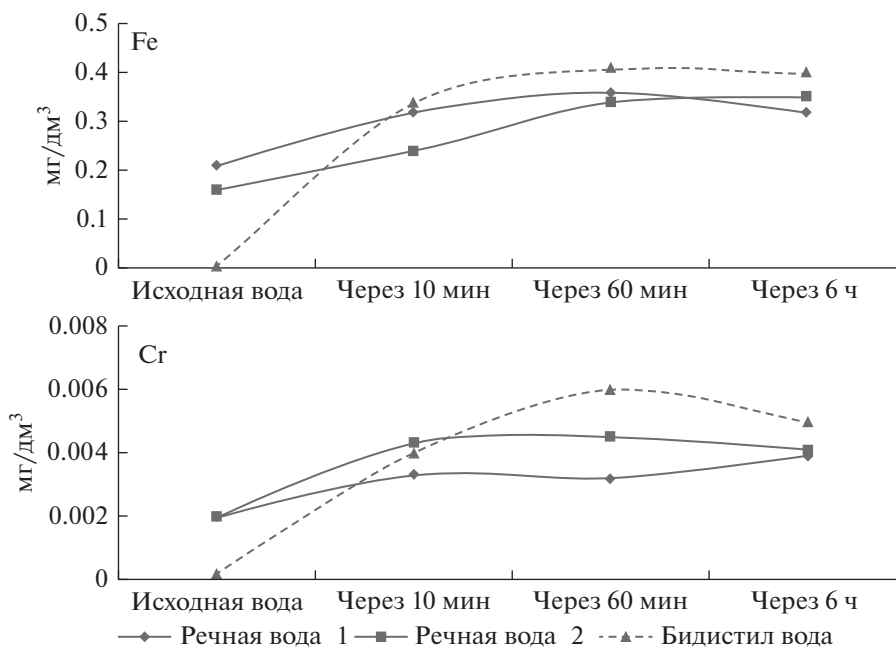
Рис. 2. Изменчивость содержания соединений железа и хрома в воде до и после эксперимента (здесь и на рис. 3: речная вода № 1 — из р. Большой Несветай; речная вода № 2 — из р. Аюта, более минерализованная).
