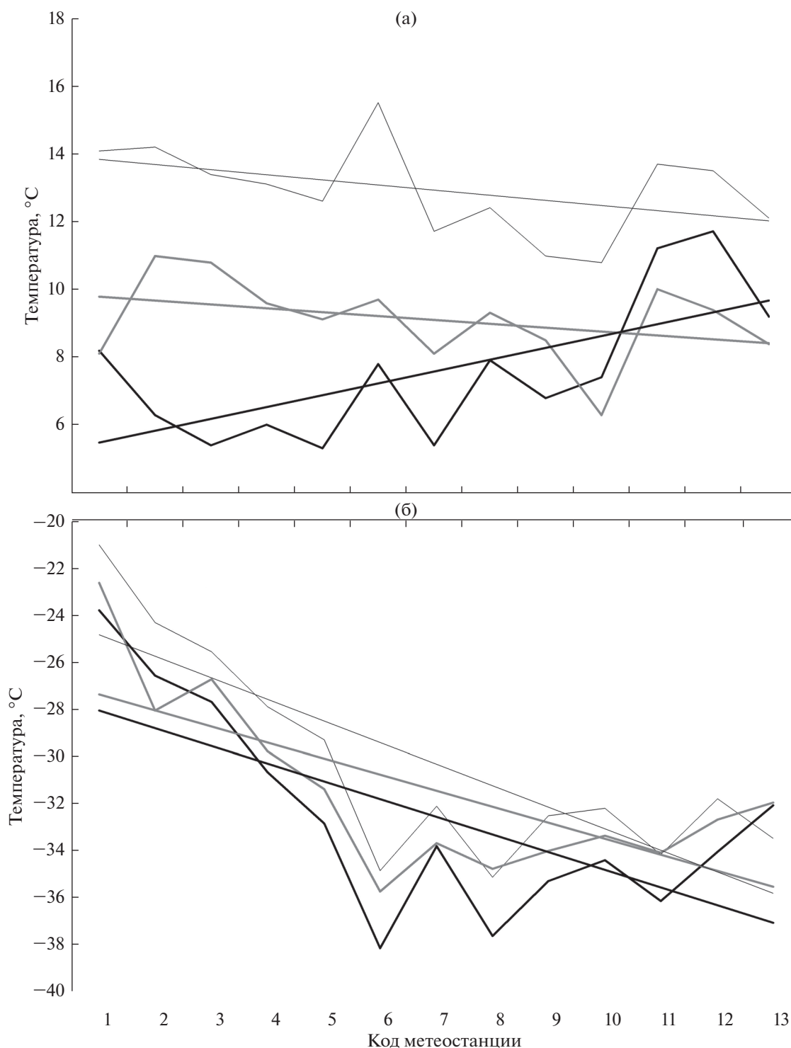
Рис. 2. Ход температуры и тренды летнего (а) и зимнего (б) периодов: июнь и январь (черная линия), июль и февраль (темно-серая линия), август и декабрь (светло-серая линия).
