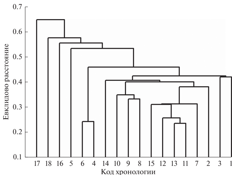
Рис. 6. Кластерный анализ коэффициентов корреляции хронологий светлых колец лиственницы с температурой воздуха в сибирской лесотундре. 1–18 — точки отбора образцов (см. рис. 1).
