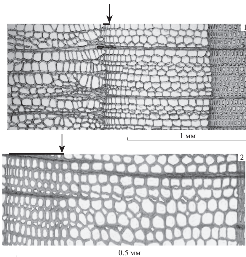
Рис. 4. Основные проявления светлых колец у лиственницы в Сибирской Субарктике. Стрелка указывает на начало поздней древесины. Увеличение \times 400 .
