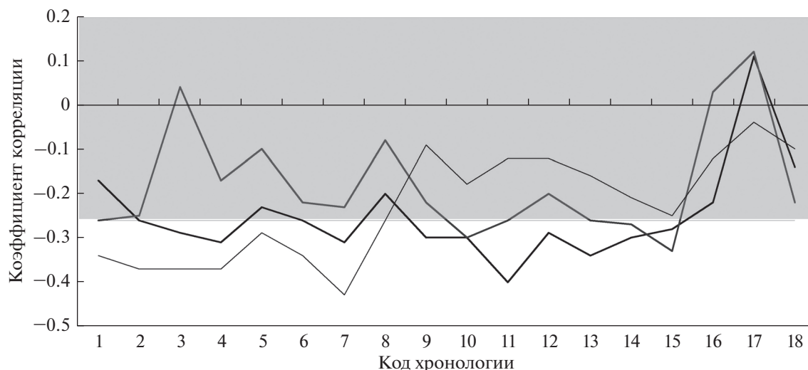
Рис. 5. Корреляции между температурой июня (черная линия), июля (серая линия) и августа (тонкая линия) и хронологиями светлых колец. Заливка серым — статистически недостоверные значения, на белом фоне — значимые коэффициенты, p < 0.05 . 1–18 — точки отбора образцов (см. рис. 1).
