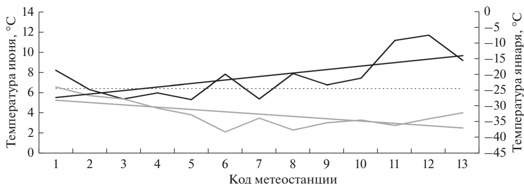
Рис. 3. Амплитуда температуры января (серая линия) и июня (черная линия). Пунктирная линия — средняя температура июня (без станций 11–13).
