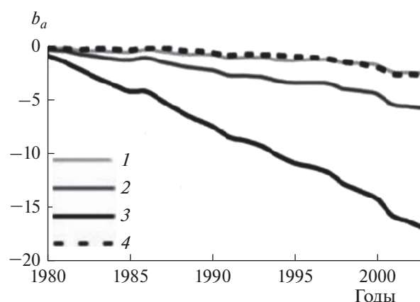
Рис. 2. Измерение и моделирование кумулятивного баланса массы b_a ледника Девон, в м водного эквивалента год -1 , источник (Gardner, Sharp, 2009): 4 — измеренный b_a ; 3 — моделирование b_a с использованием влажноадиабатического градиента температуры воздуха \gamma = -6.58^\circ\text{C км}^{-1} ; 2 — моделирование b_a по данным измерений градиента \gamma = -4.98^\circ\text{C км}^{-1} ; 1 — в модели b_a использован расчет \gamma в зависимости от температуры воздуха в опорном пункте.
