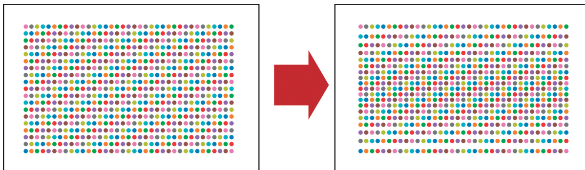
Рис. 2. Пересчет географических координат (долгота/широта) в проекцию Голла.
