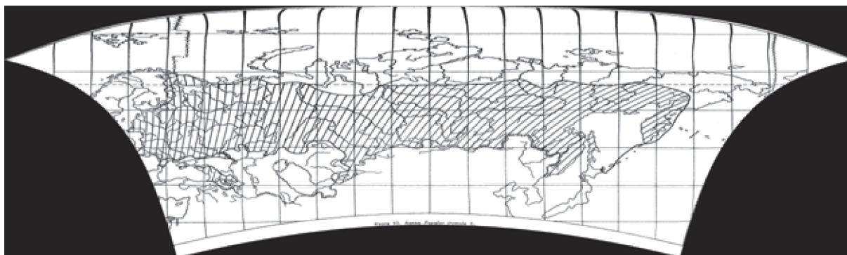
Рис. 6. Ареал Populus tremula L в координатах долгота/широта.
