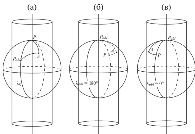
Рис. 3. Поворот сферы относительно цилиндра для перехода к географическим координатам в косо́й ориентировке.
