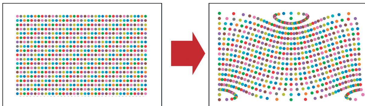
Рис. 4. Переход от нормальной (широта/долгота) к косо́й ориентировке.
