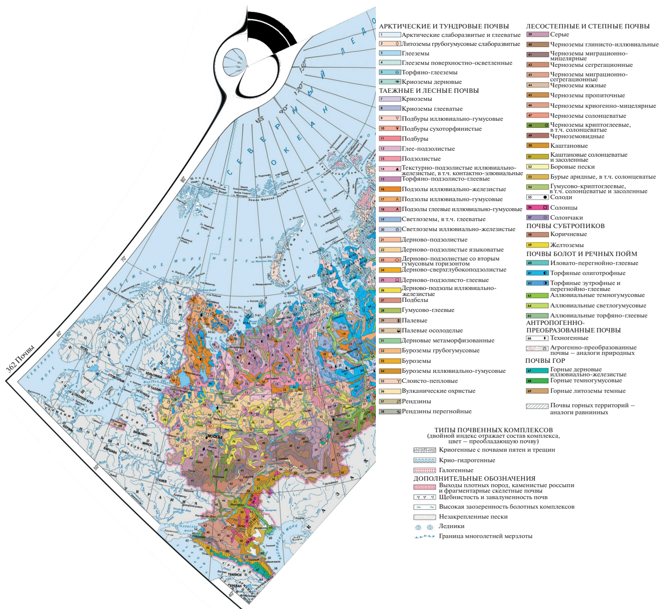
Рис. 5. Фрагмент почвенной карты после трансформирования в проекцию Красовского.
