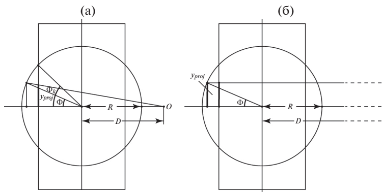
Рис. 1. Перспективно-цилиндрическая проекция в нормальной ориентировке с различным расстоянием от точки глаза.
