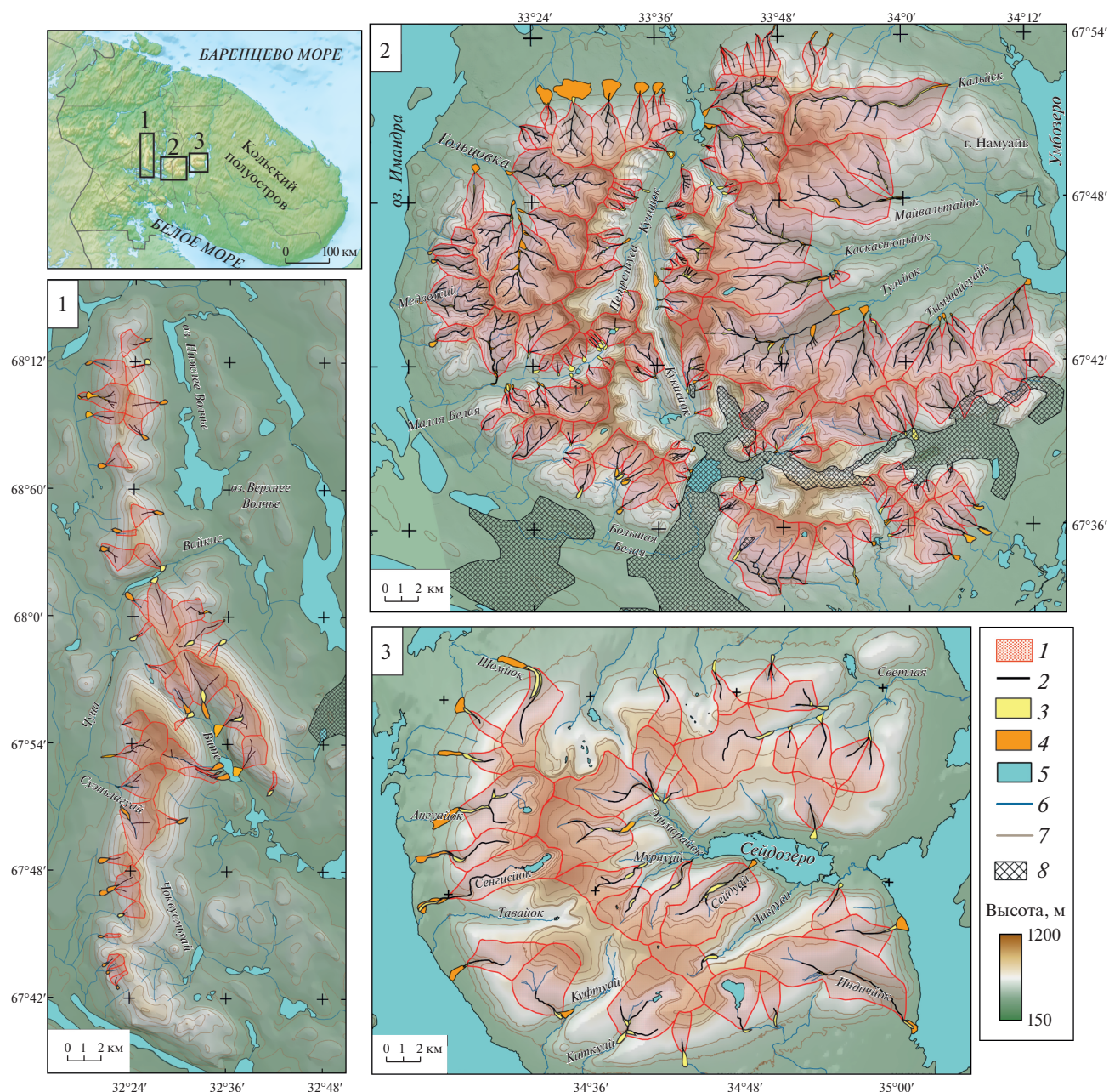
Рис. 1. Селевые бассейны гор Кольского полуострова (1 – Монче-, Чуна- и Вольчи тундры, 2 – Хибины, 3 – Ловозерские тундры).
