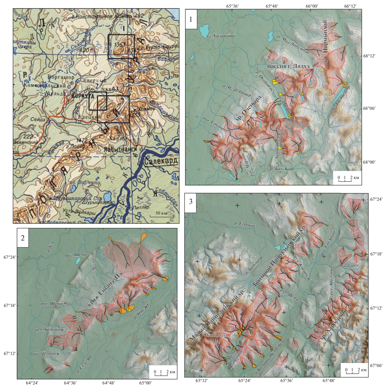
Рис. 2. Селевые бассейны ключевых участков Полярного Урала (1 — хр. Оченырда, массив г. Лядхэ, хр. Нармынхой, 2 — кряж Енганепэ, 3 — Малый Пайпудынский, Большой Пайпудынский, Харбейский хребты). Условные обозначения см. на рис. 1.
